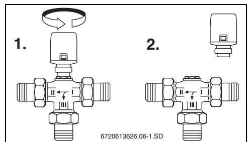
Fig. 10 Demontați servomotorul.
