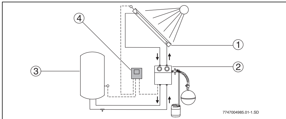
Fig. 2 Schemă instalație
